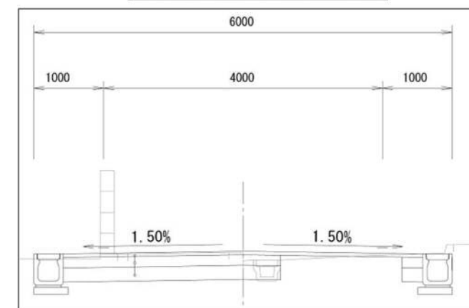
標準断面図（A-A 断面）
