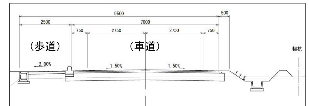
標準断面図（A-A断面）
