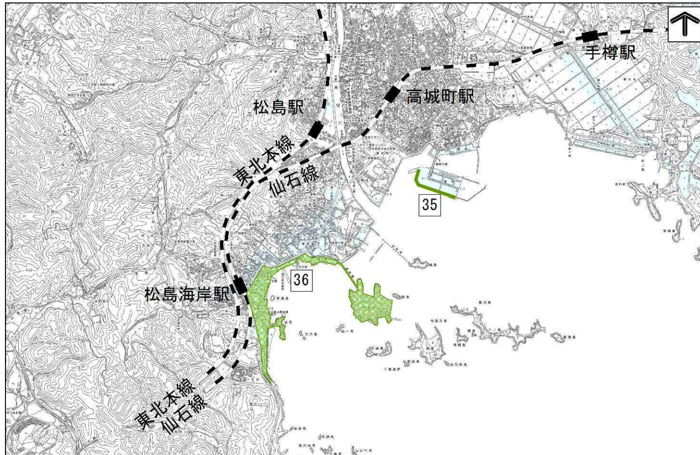
■計画平面図
