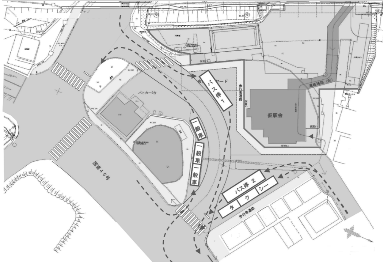
松島海岸駅 駅前広場仮設計画図
