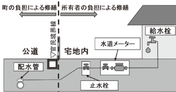
給水装置修繕に係る費用負担の図 ※宅地内の給水装置の修繕は、所有者の負担となります。
